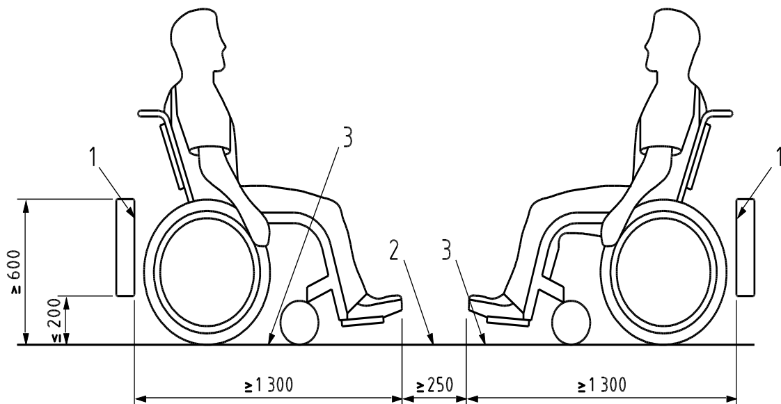
Abb. I3: Zwei Vis-à-vis-Rollstuhlplätze
