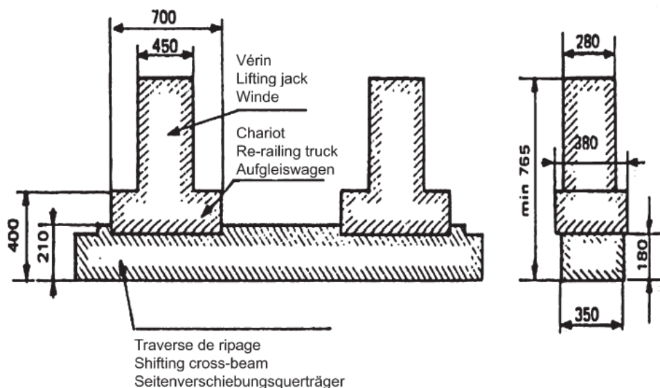
Aufgleisung / Rerailing / Relevage sur la voie
