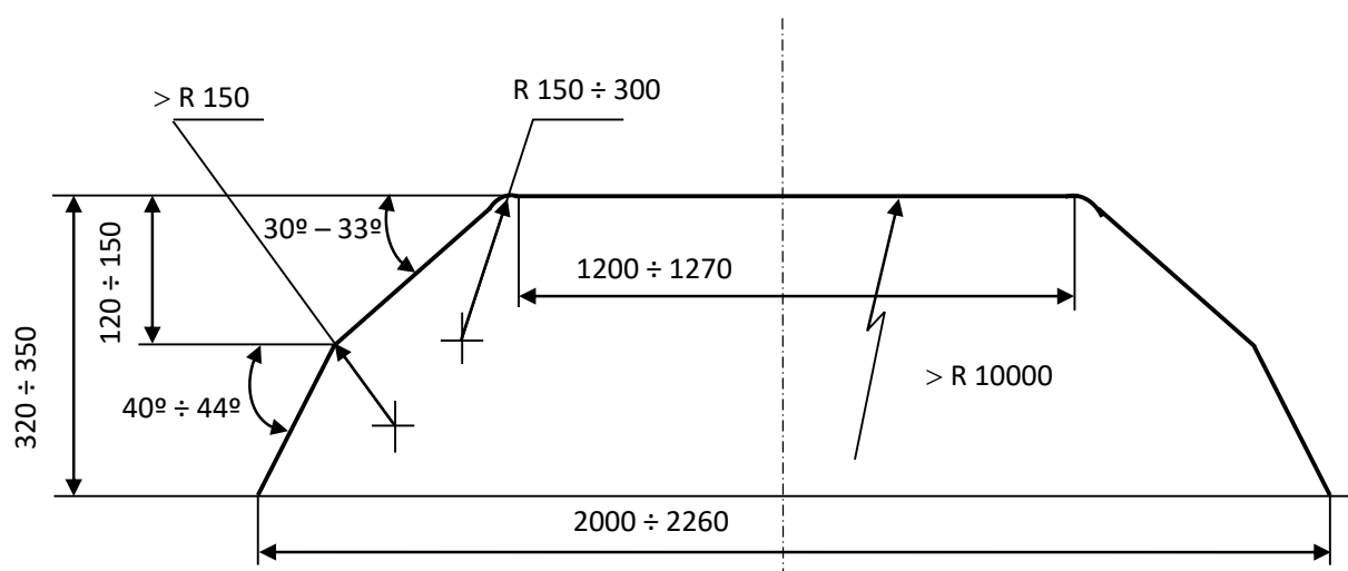
Figure : Configuration et dimensions des archets
