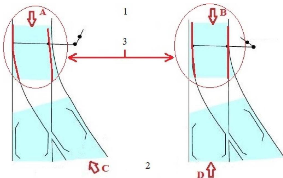
Figure K.3 : Mesure de déplacement de l'aiguillage
