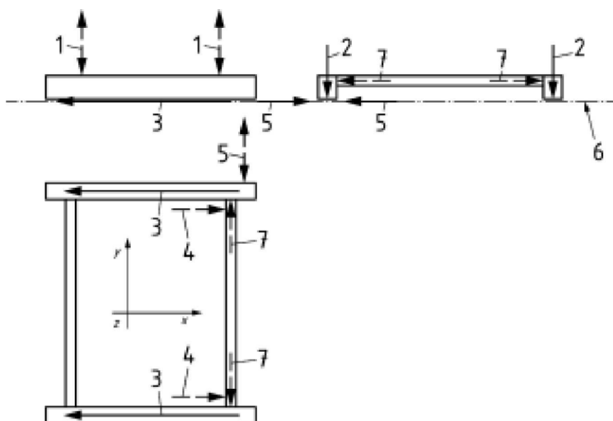
Abbildung K.2 Überblick über die Kraftübertragung
