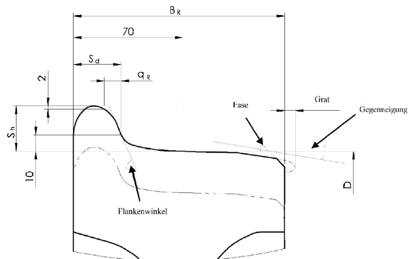
Abbildung 2. Bezeichnungen für Räder
