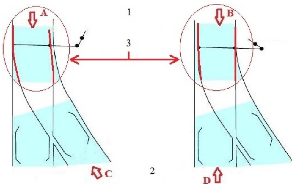
Abbildung K.3 Messung der Verschiebung der Weiche
