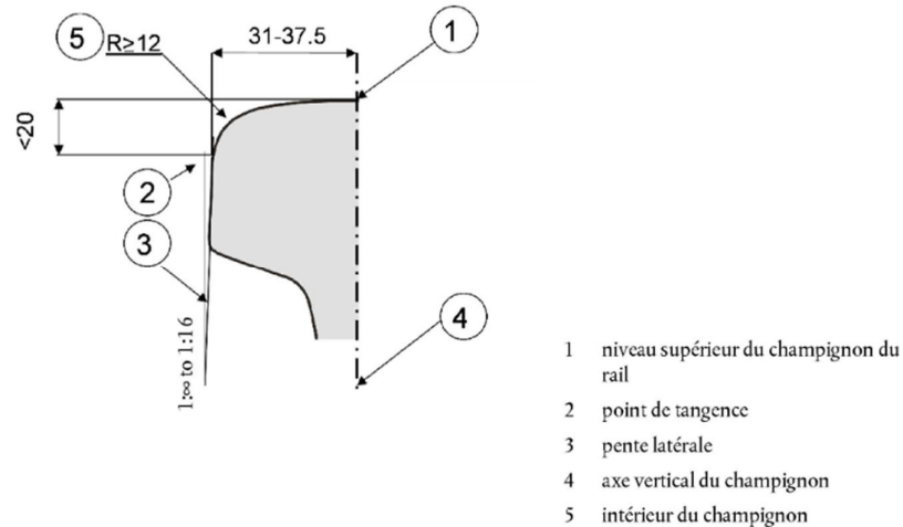
Figure 1 : Profil du champignon de rail
