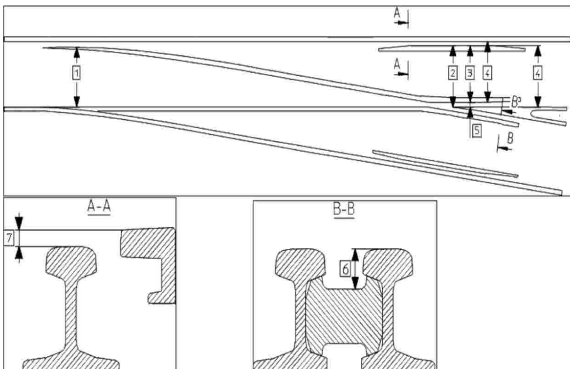
Figure 14 : Géométrie des appareils de voie
