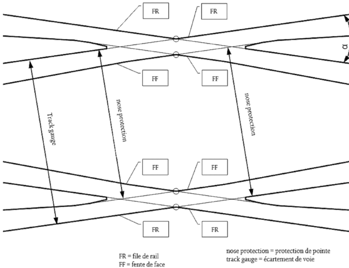
Figure 6 : Traversée avec lacune
