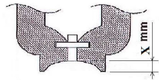
Abbildung K.1 Höchstzulässiger Hohllauf
