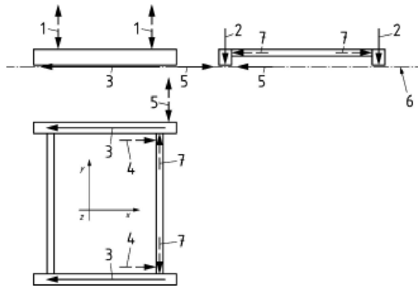
Abbildung K.2 Überblick über die Kraftübertragung
