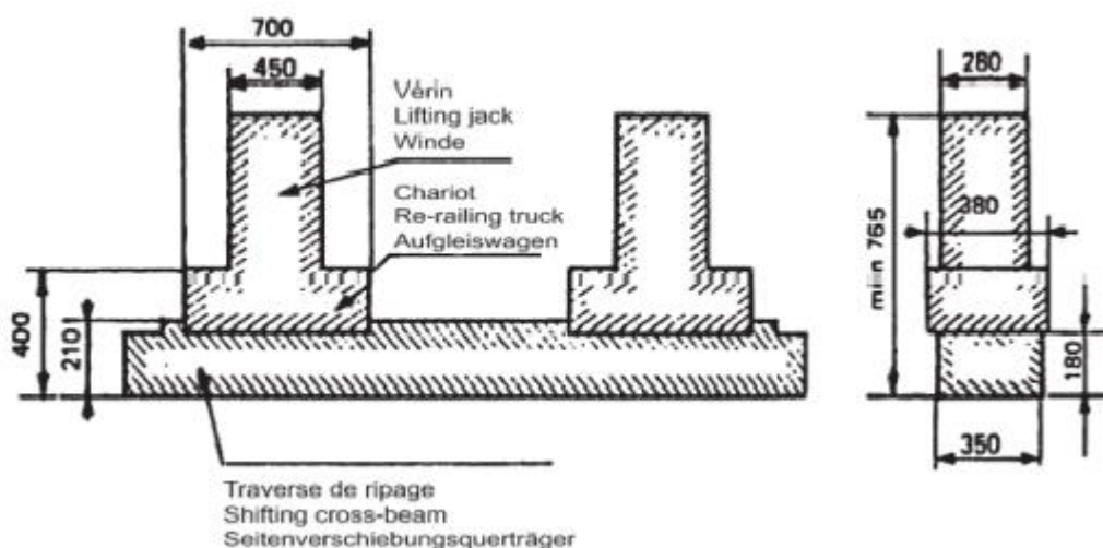
Freier Raum unter Aufgleisstellen
