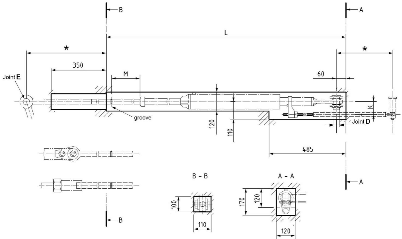
Abb. 1: Hüllräume bei Lasten bis maximal 75 kN
