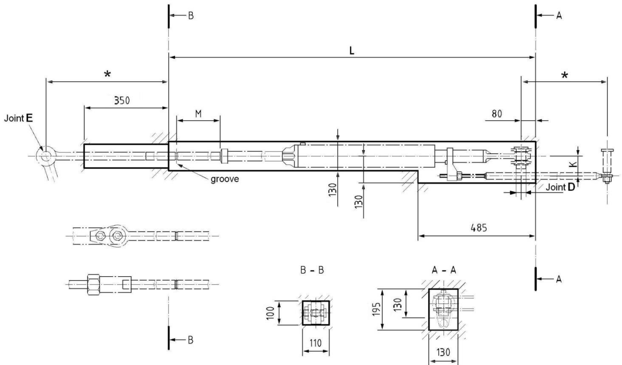
Abb. 2: Hüllräume bei Lasten über 75 kN
