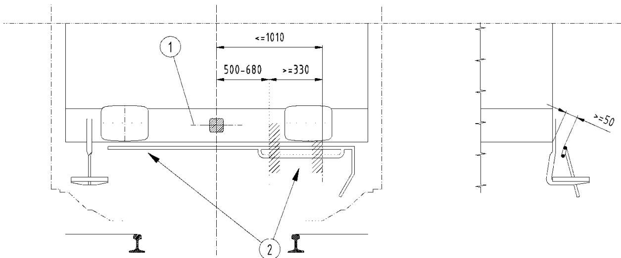
Figure 8 : Position des mains courantes d'attieur en cas d'utilisation d'un attelage automatique
