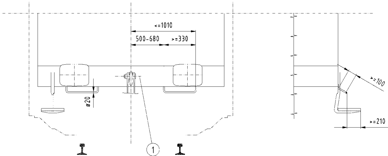
Figure 7 : Positions des mains courantes d'attieur
