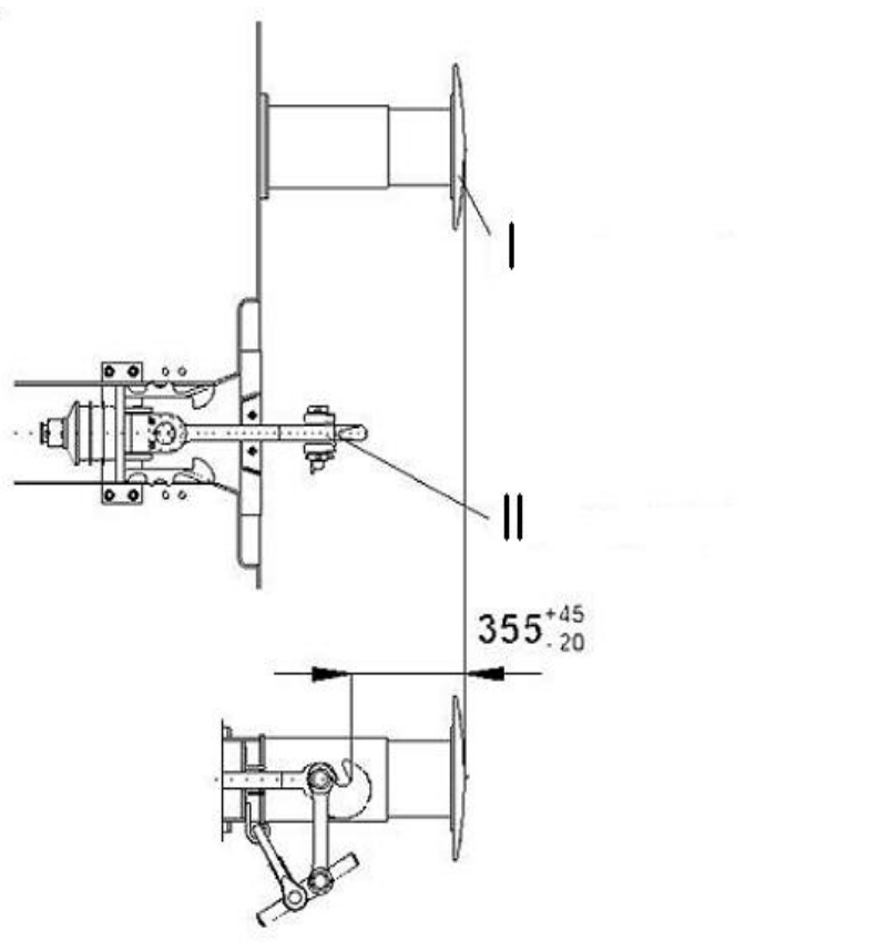
Illustration A1 Organes de choc et de traction
