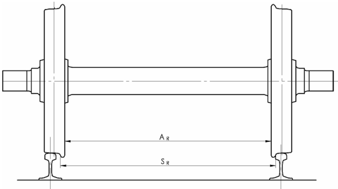
Illustration 1. Symboles utilisés pour les essieux montés
