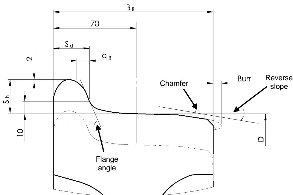
Illustration 2. Symboles utilisés pour les roues
