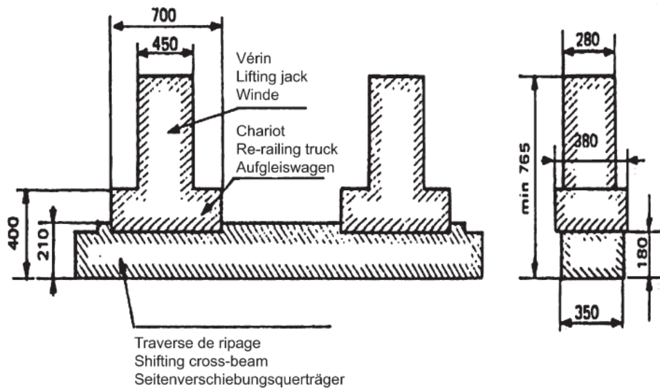
Rerailing / Relevage sur la voie
