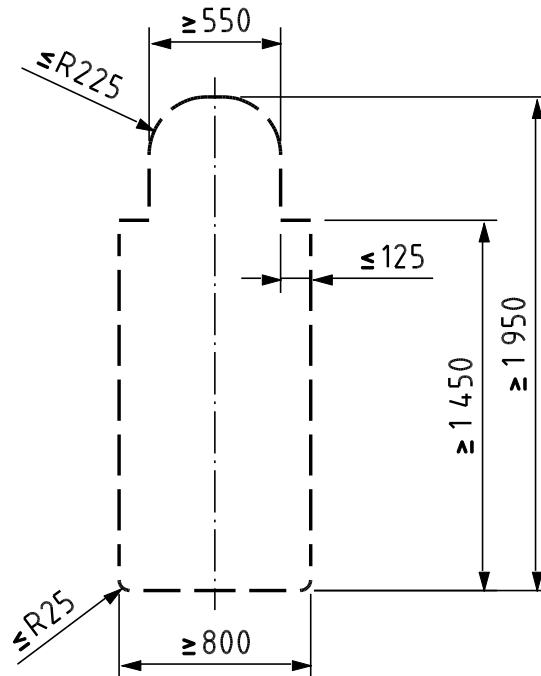
Abb. J3: Mindestlichraum der Verbindungen zwischen Rollstuhlplätzen
