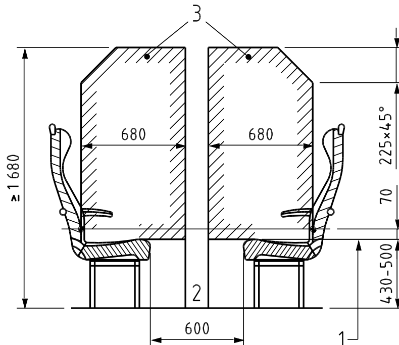
Abb. H2: Behindertensitze in Reihenordnung
