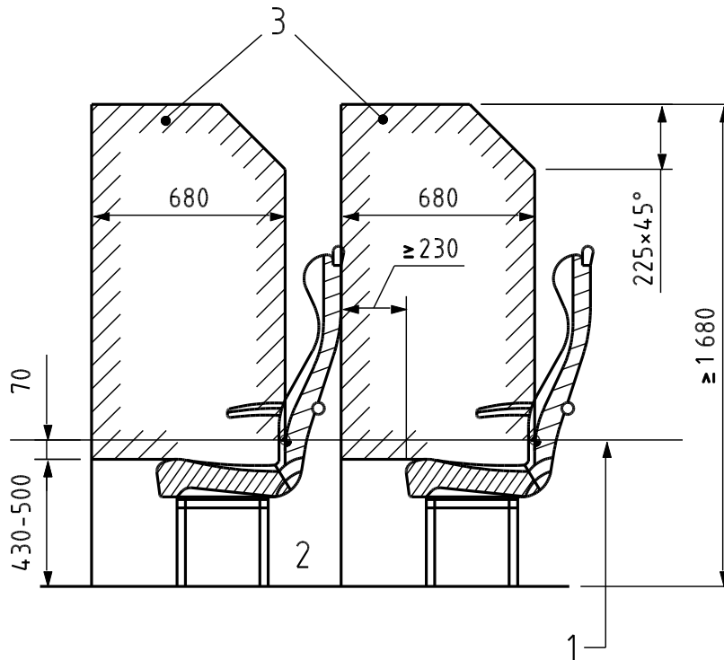
Abb. H2: Behindertensitze in Reihenordnung
