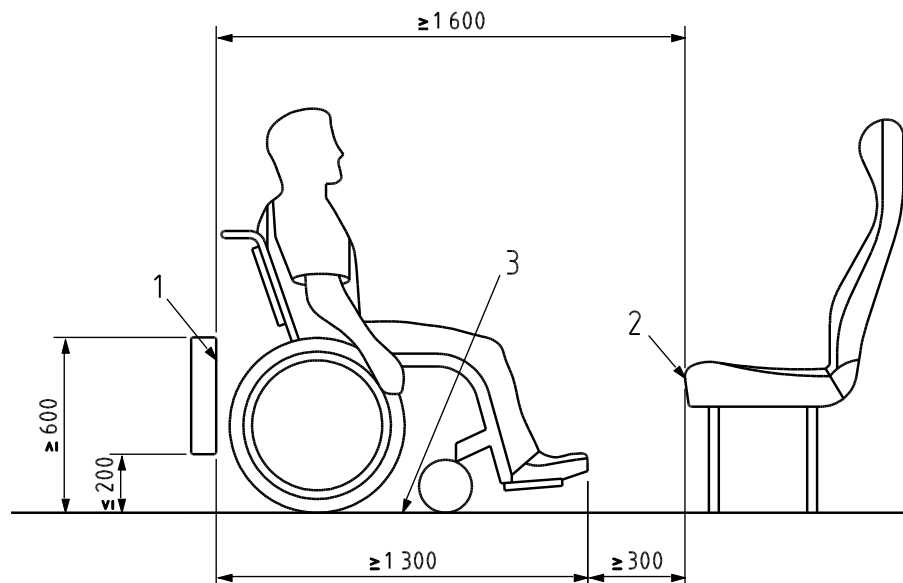
Abb. I1: Rollstuhlplatz mit Vis-à-vis-Sitzanordnung
