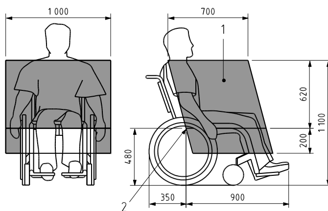
Abb. L1: Reichweite von Rollstuhlfahrern
