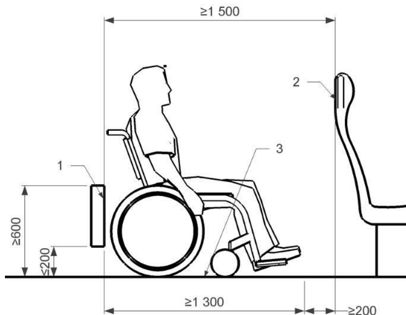
Abb. I2: Rollstuhlplatz in Reihenordnung
