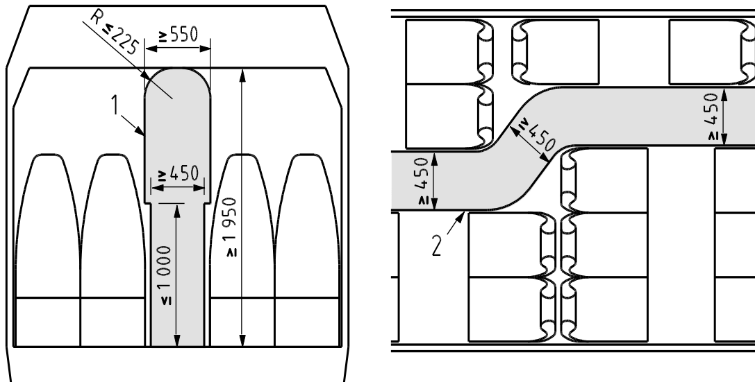
Abb. J1: Mindestbreite des lichten Raums vom Boden bis zu einer Höhe von 1000 mm
