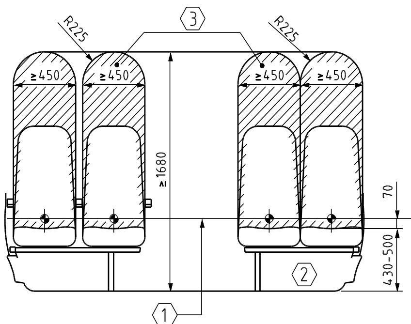
Abb. H1: Lichte Höhe über den Behindertensitzen
