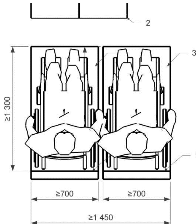
Abb. I4: Zwei nebeneinander angeordnete Rollstuhlplätze (gilt nur für umgerüstete/erneuerte Fahrzeuge)
