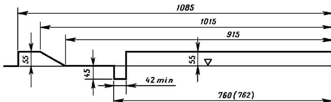
Figure 4 Contour de référence des pièces inférieures sur les voies équipées d'une traversée-jonction double
