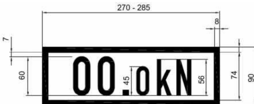
Abbildung- 3: Kennzeichnung-Anschrift der Bremskraft der Feststellbremse
