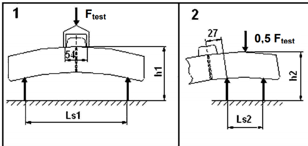
Abbildung-Abb. 3: Aufbau für die Prüfung der Biegefestigkeit
