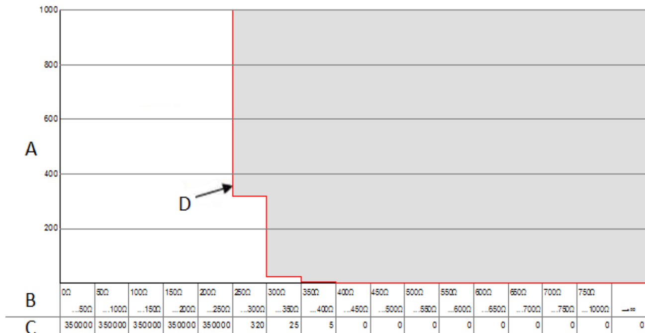
Abbildung Abb. 9: Grenzwerte pro Impedanzklasse für kontaminierte Bremscheiben
