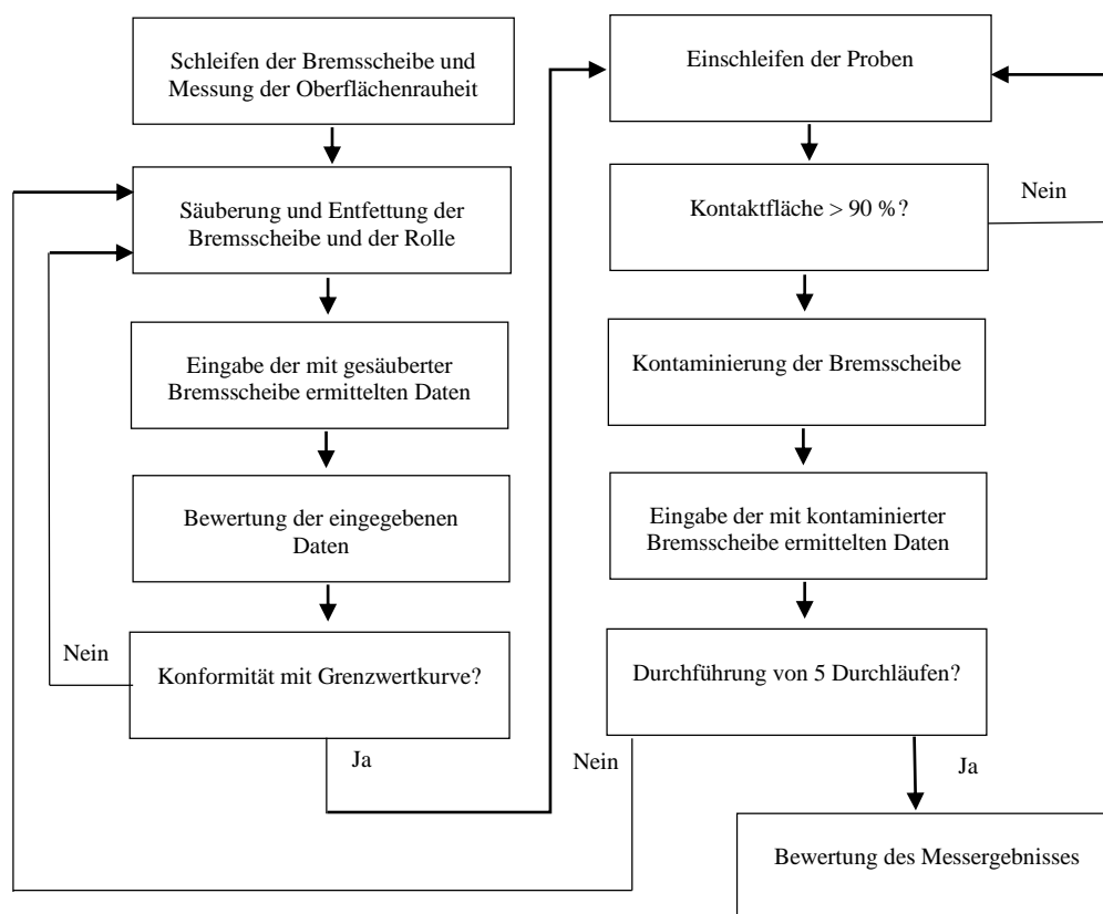
Abbildung-Abb. 4: Ablaufdiagramm des Prüfprogramms
