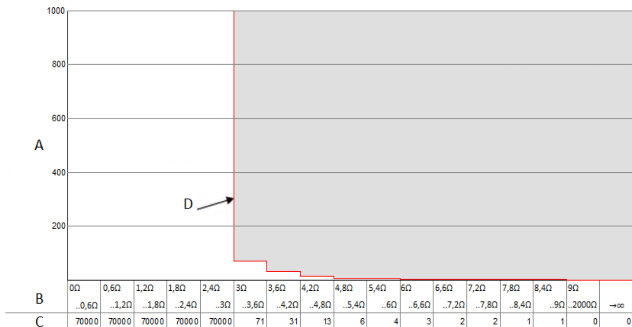
Abbildung Abb. 8: Grenzwerte pro Impedanzklasse für gesäuberte Bremsscheiben
